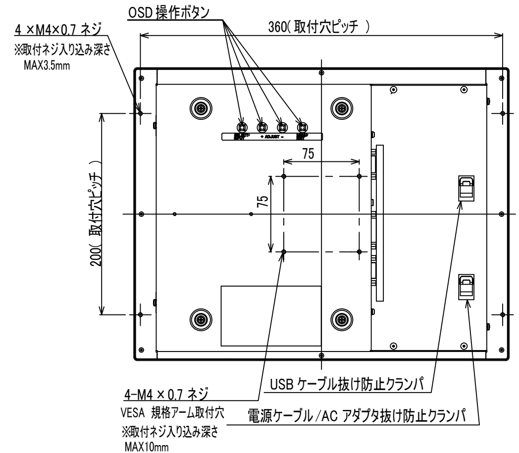
パネル取付穴推奨図
