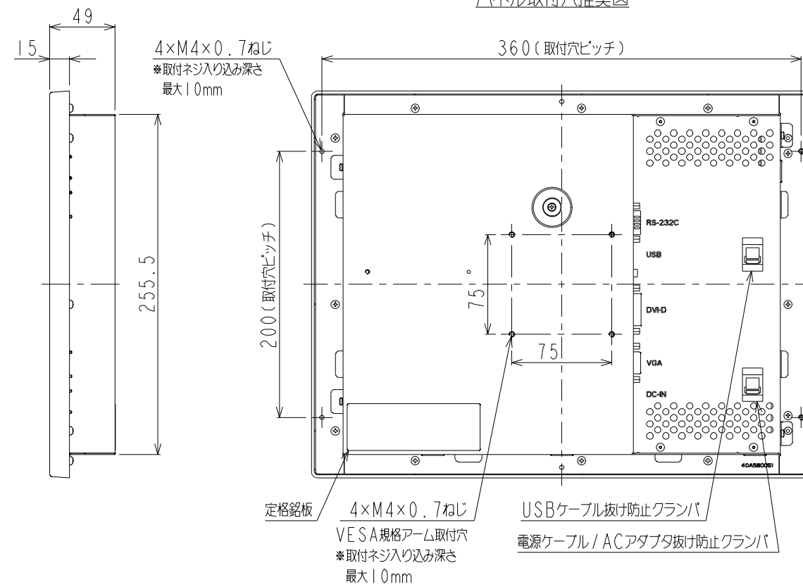
パネル取付穴推奨図
