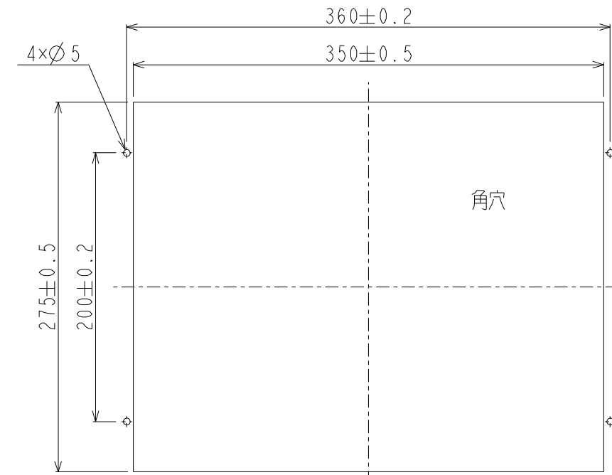
パネル取付穴推奨図
