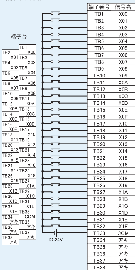
外部接続図(例)
