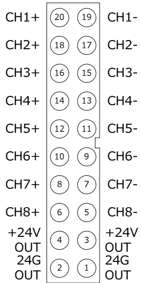
信号出力用コネクタ CON1, CON2 コネクタピン配置図 (Top view)
