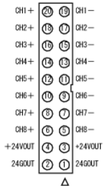
信号入出力用コネクタ CON1、CON2 コネクタピン配置図 (TOP VIEW)
