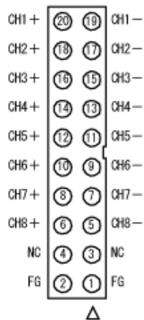
信号出力用コネクタ CON1, CON2 コネクタピン配置図 (TOP VIEW)
