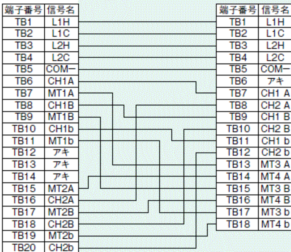
A1S64TCTRT (加熱冷却制御、白金測温抵抗体) 端子台
