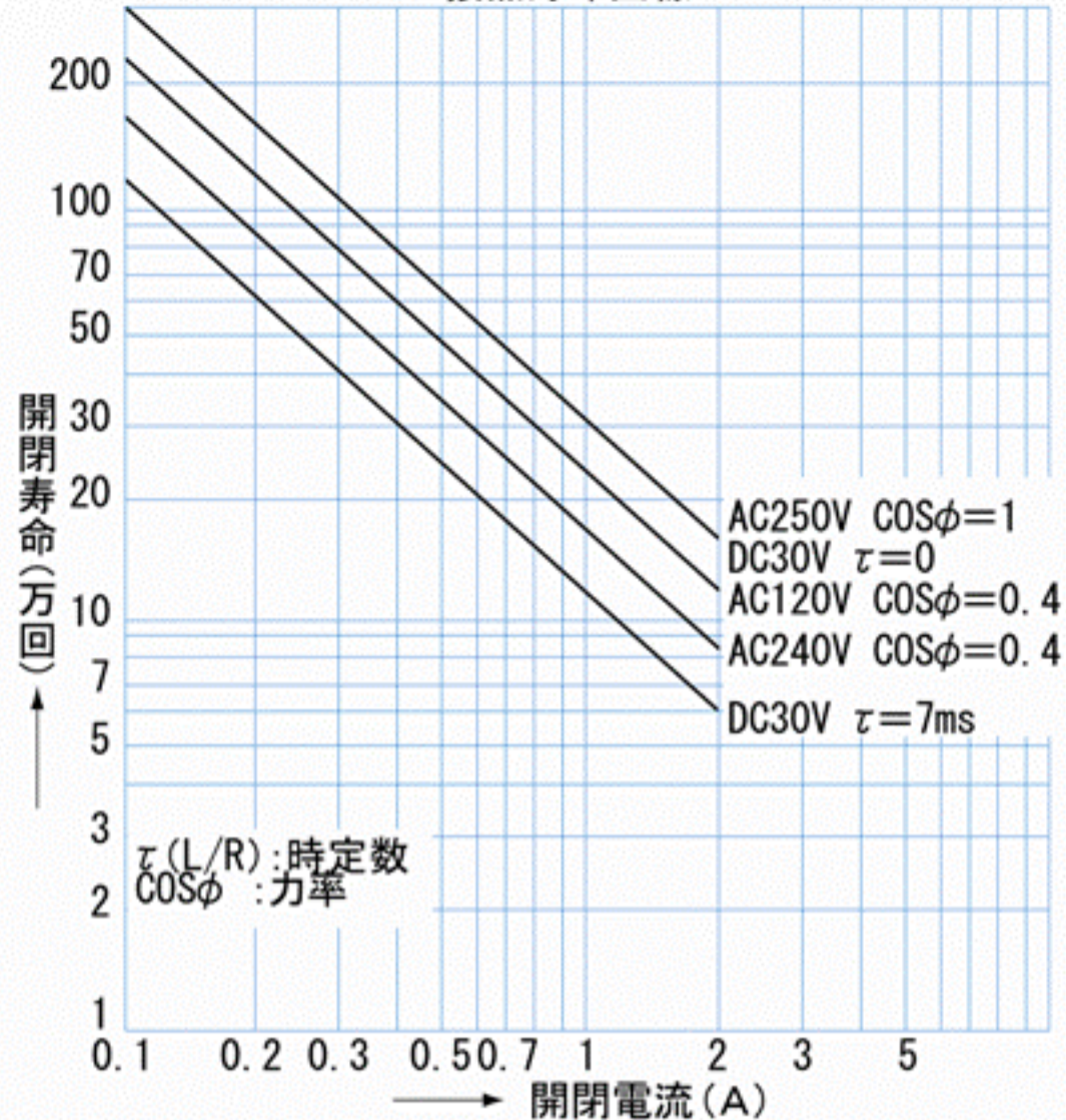
b接点寿命曲線
