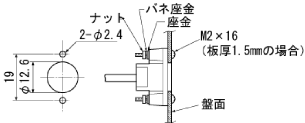
盤面取付穴参考寸法および取付寸法(参考)
