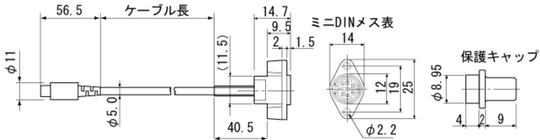
盤面取付穴参考寸法および取付寸法(参考)
