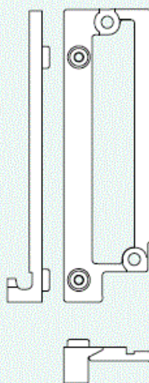
取付板
