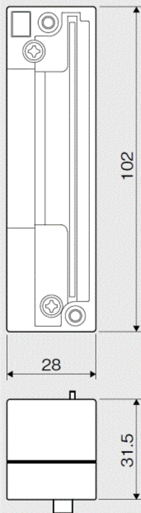
変換アダプタ
