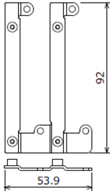
取付金
