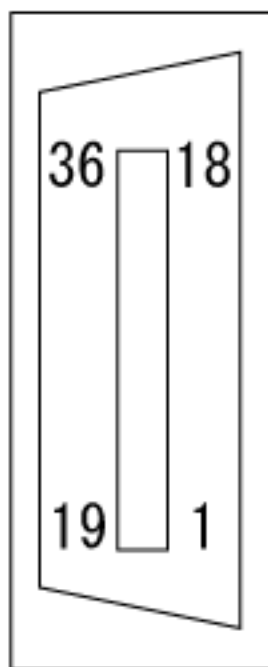
A1SD75P□-S3コネクタ向き (TOP VIEW)
