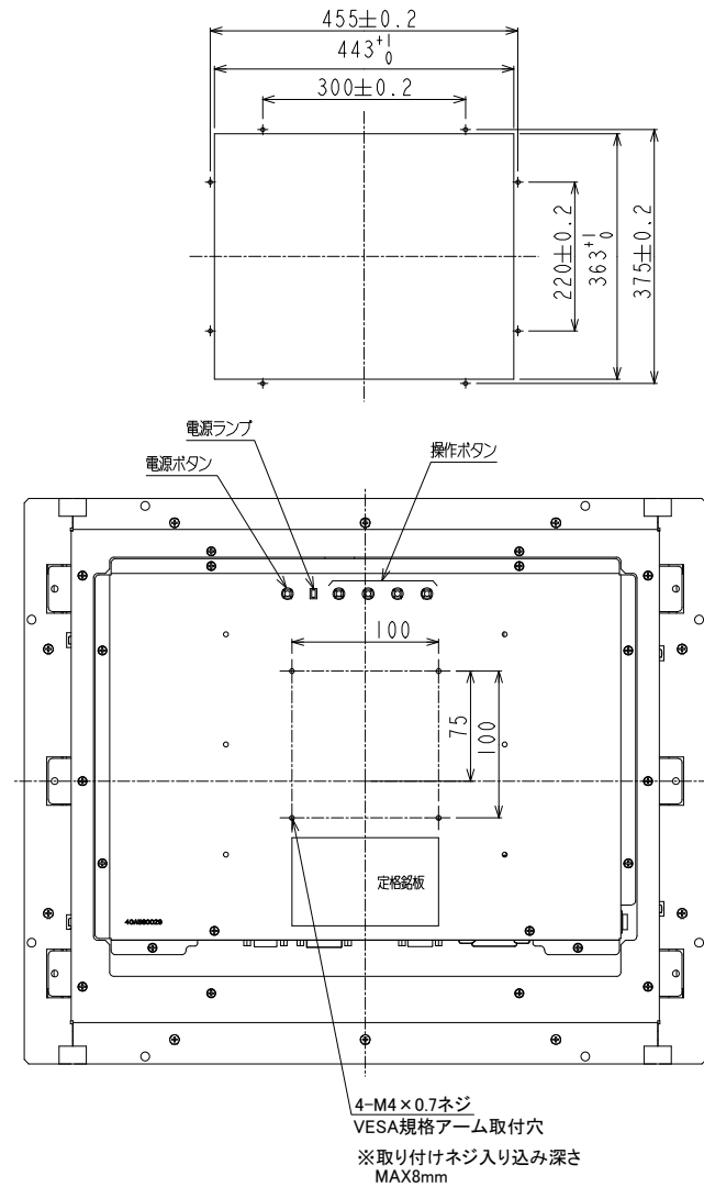
パネル取付穴推奨図
