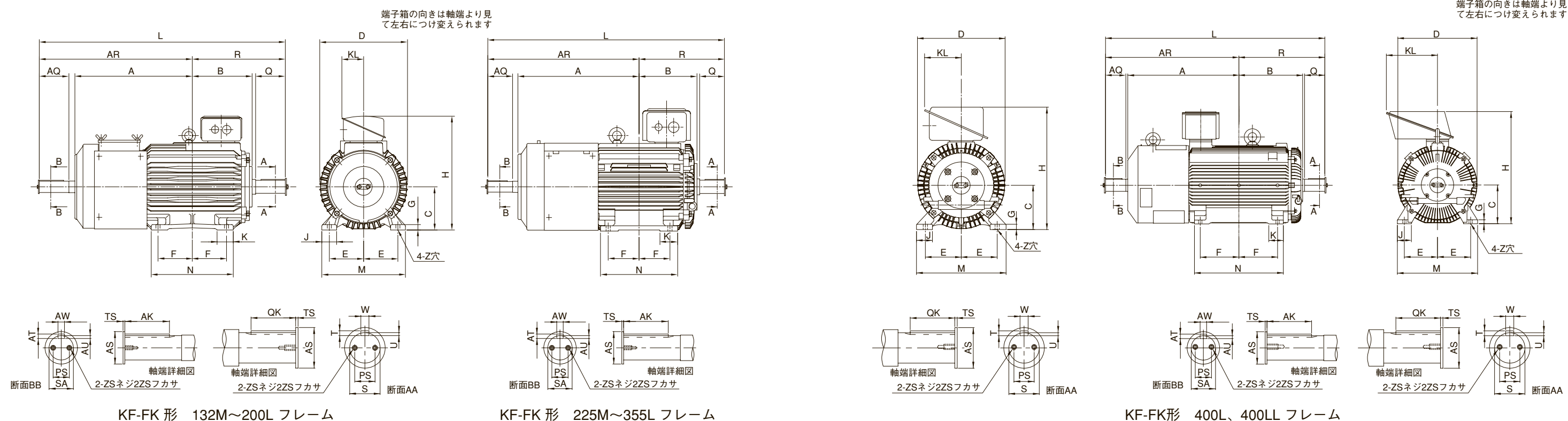
図4 KF-FK形クレーン用三相誘導電動機外形寸法図
