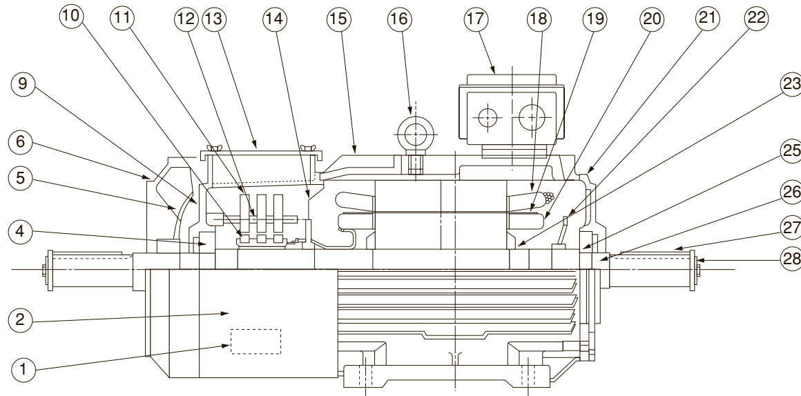
図3-1 KF-FK 160Lフレームの場合
