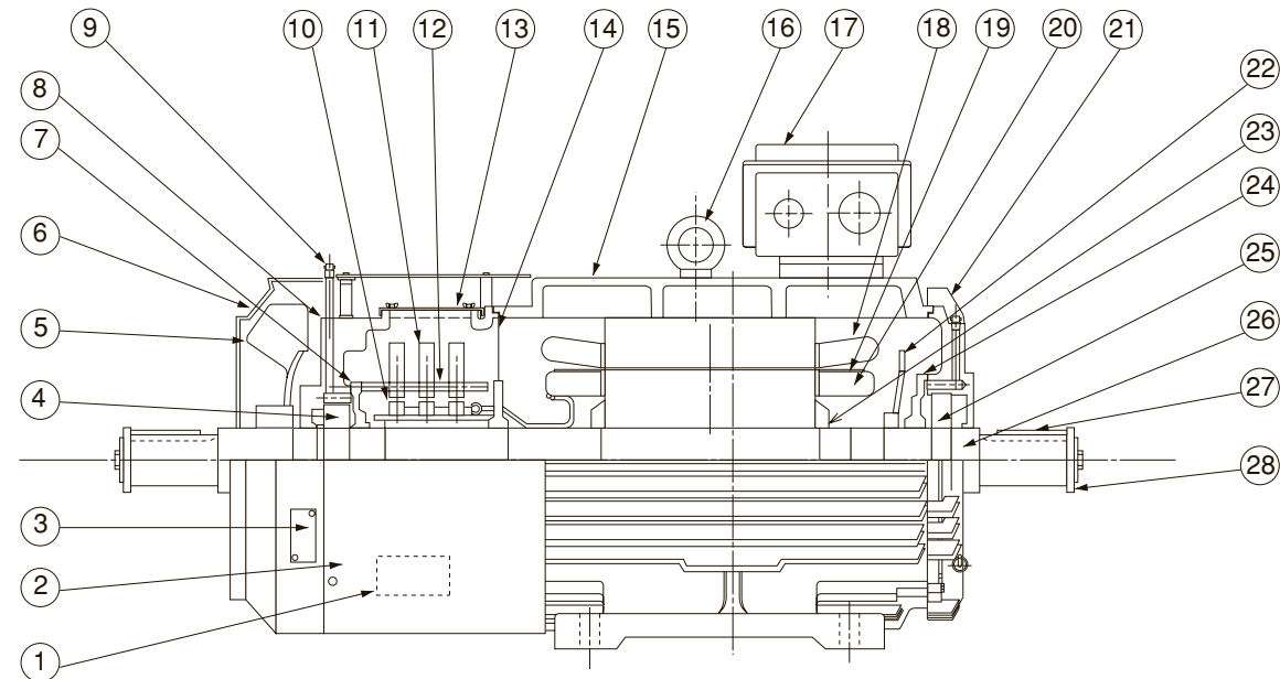
図3-2 KF-FK 315Mフレームの場合
